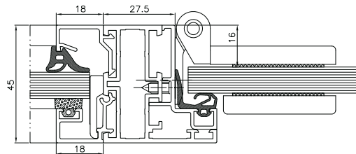
Querschnitt durch den Pfosten
