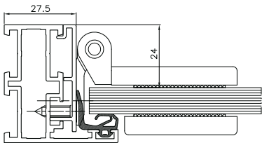
Seitlicher Querschnitt der Tür
